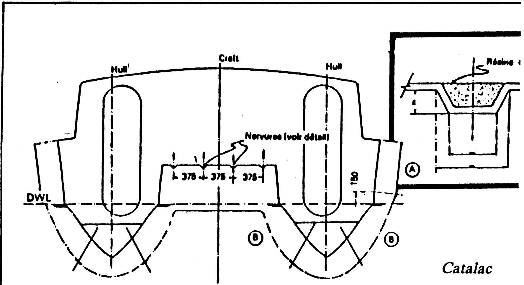
coupe au maître couple (C) Chatenay 1977
